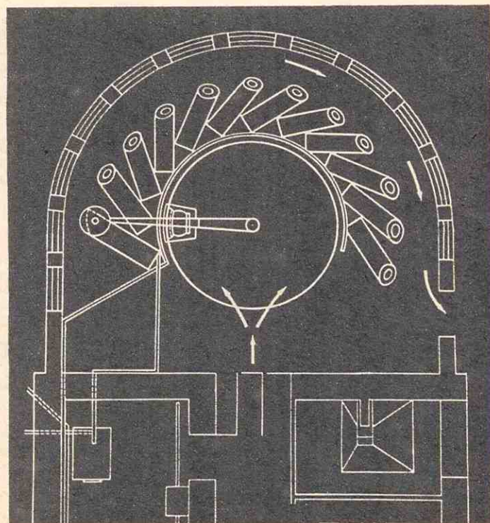
План доильной установки.
